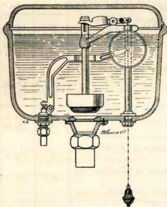
Coupe du Réservoir N° 4162.
